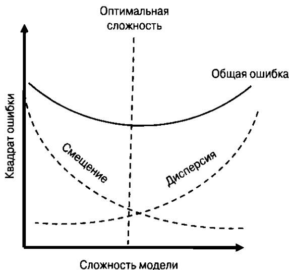
Рис. 4.3. Обычно достижением компромисса между смещением и дисперсией удается найти точку оптимальной сложности модели
