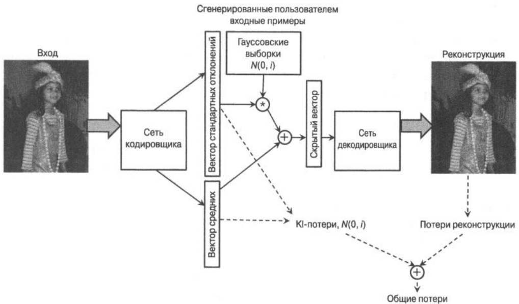
Рис. 4.12. Репараметризация вариационного автокодировщика
