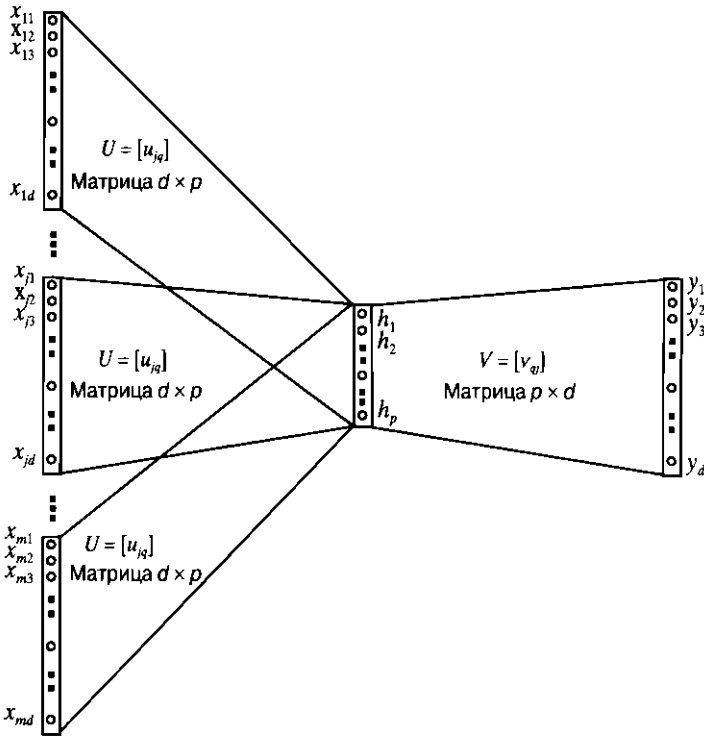
Рис. 2.15. Word2vec: модель SBoW. Обратите внимание на то, в чем этот рисунок сходен, а в чем отличается от рис. 2.13, соответствующего единственному набору входов и линейному выходному слою. Того же результата можно было бы добиться, свернув t наборов, состоящих из d входных узлов каждый, в единственный набор, состоящий из d входов, и агрегировав t входов в представлении прямого кодирования в одном окне. В этом случае вход уже не будет представлен прямыми кодами
