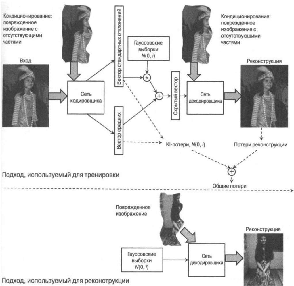
Рис. 4.15. Восстановление поврежденных изображений с помощью условного вариационного автокодировщика. Данные изображения использованы исключительно в иллюстративных целях
