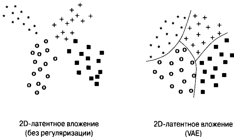
Рис. 4.14. Распределенные представления, созданные вариационным автокодировщиком и нерегуляризованной версией автокодировщика. Нерегуляризованная версия характеризуется наличием больших разрывов в латентном пространстве, которые могут не соответствовать значимым точкам. В случае вариационного автокодировщика гауссовское распределенное представление делает возможным семплирование
