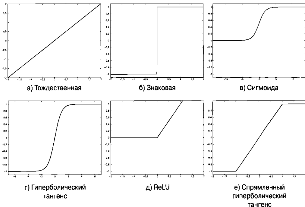
Рис. 1.8. Разновидности функции активации
