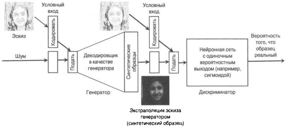
Рис. 10.10. Условная генеративно-сопоставительная сеть для подключенного дискриминатора. Поучительно сравнить эту архитектуру с архитектурой безусловной генеративно-сопоставительной сети, приведенной на рис. 10.7
