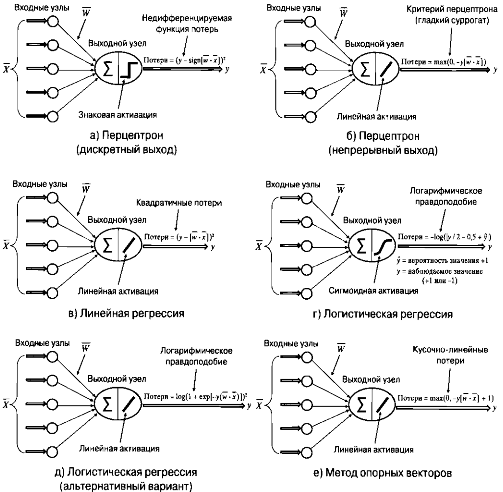
Рис. 2.3. Различные варианты перцептрона
