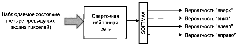
Рис. 9.6. Сеть стратегий, соответствующая условиям видеоигр на платформе Atari. Понятно сравнить эту конфигурацию с Q-сетью, представленной на рис. 9.3
