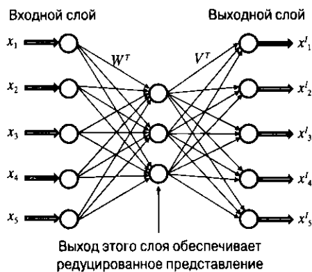
Рис. 2.7. Базовый автокодировщик с одним слоем
