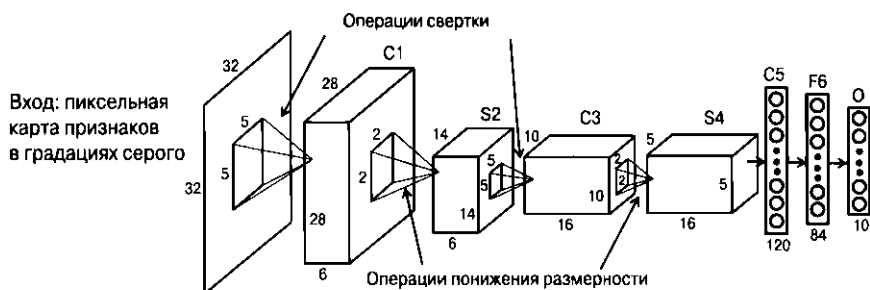
а) Детальное представление архитектуры
