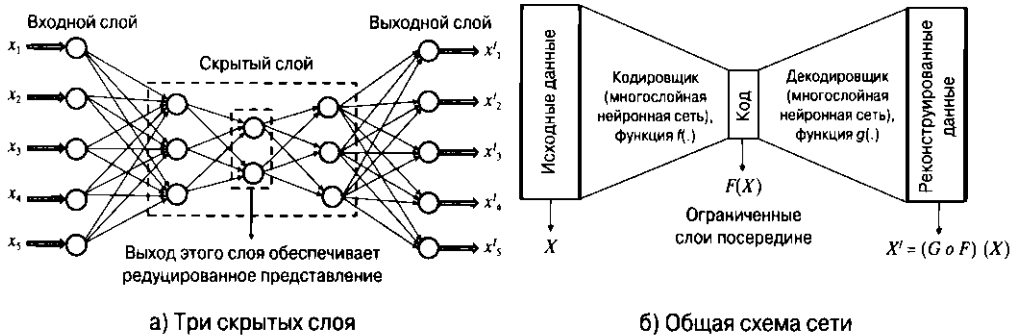
Рис. 2.6. Базовое схематическое представление автокодировщика
