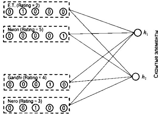
б) Архитектура RBM для Боба (наблюдаемые рейтинговые оценки: E.T. , Nixon , Gandhi и Nero )
