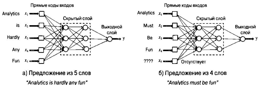
Рис. 7.1. Попытки использования обычной нейронной сети для sentiment-анализа наталкиваются на трудности обработки входов переменной длины. Архитектура сети также не содержит никакой полезной информации о зависимостях, обусловленных порядком следования слов
