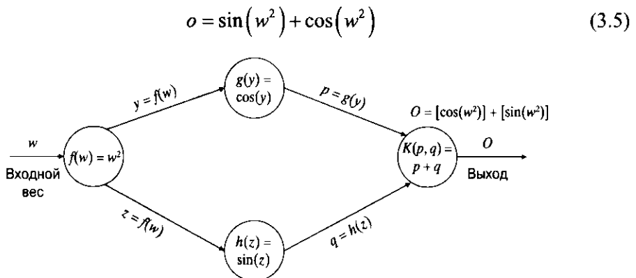
Рис. 3.3. Пример применения цепного правила на основании вычислительного графа, приведенного на рис. 3.2
