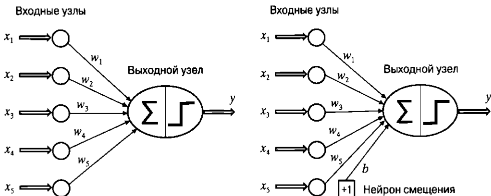
а) Перцептрон без смещения
