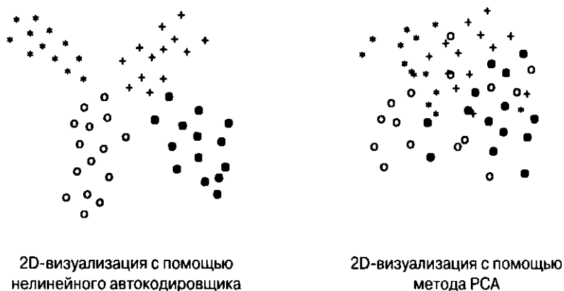
Рис. 2.11. Типичные различия между вложениями, созданными с помощью нелинейных автокодировщиков и по методу анализа главных компонент (PCA). Нелинейные и глубокие автокодировщики часто способны разделять переплетенные классовые структуры, содержащиеся в базовых данных, что невозможно в условиях ограничений линейных преобразований наподобие PCA. Это происходит по той причине, что отдельные классы часто заполняются в исходном пространстве на таких искривленных многообразиях, которые, если при этом не искривлять само пространство, выглядят смешанными при рассмотрении любого двухмерного сечения данных. Данный рисунок приведен исключительно в иллюстративных целях и не представляет никакого конкретного распределения данных
