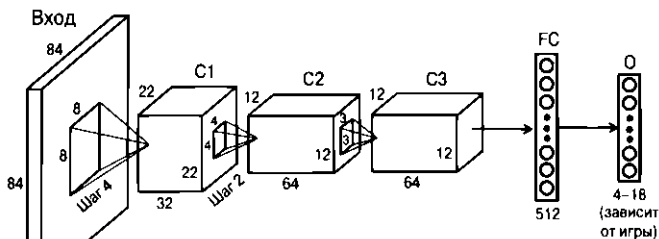
Рис. 9.4. Сверточная нейронная сеть для игр на платформе Atari
