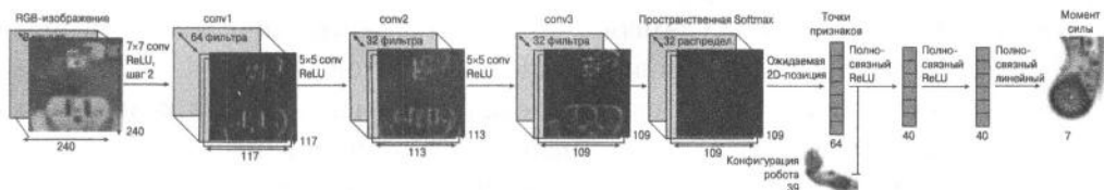
б) Архитектура сверточной нейронной сети
