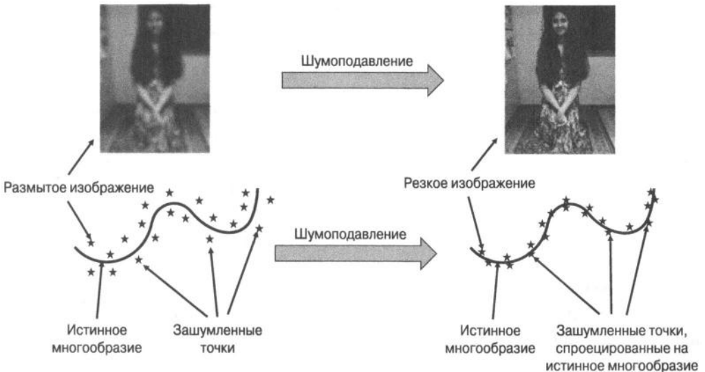
Рис. 4.10. Шумоподавляющий автокодировщик
