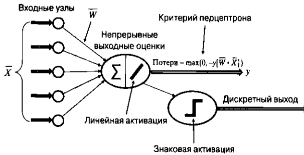
Рис. 2.2. Расширенная архитектура перцептрона с дискретными и непрерывными прогнозными значениями
